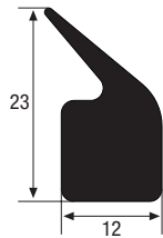
Zargenprofil
