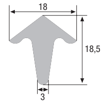
Zargenprofil
