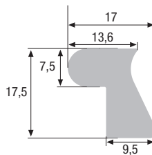
Zargenprofil
