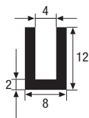
U- und Klemmpofil
