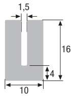
U- und Klemmprofil
