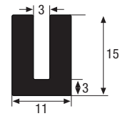
U- und Klemmprofil
