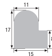
Zargenprofil
