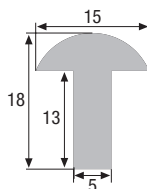
Zargenprofil
