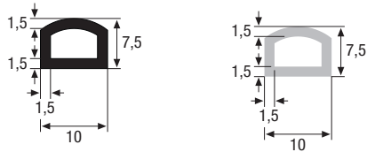
Hohlkammerprofil
