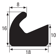
Zargenprofil
