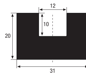
U- und Klemmprofil
