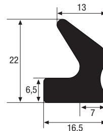
Zargenprofil
