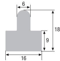
Zargenprofil
