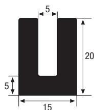
U- und Klemmprofil
