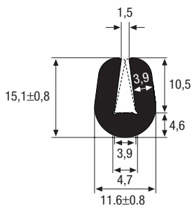
U- und Klemmprofil
